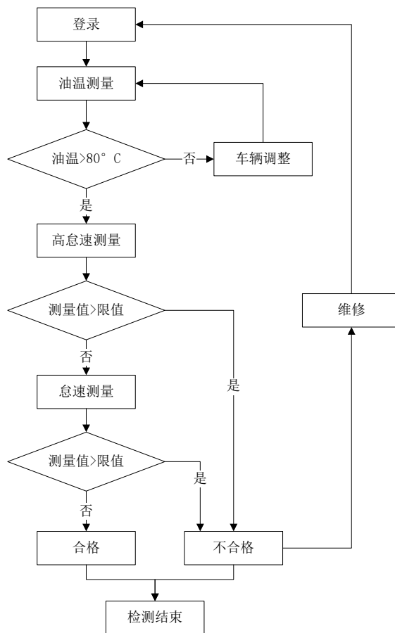
图 A.1 双怠速法测量程序
