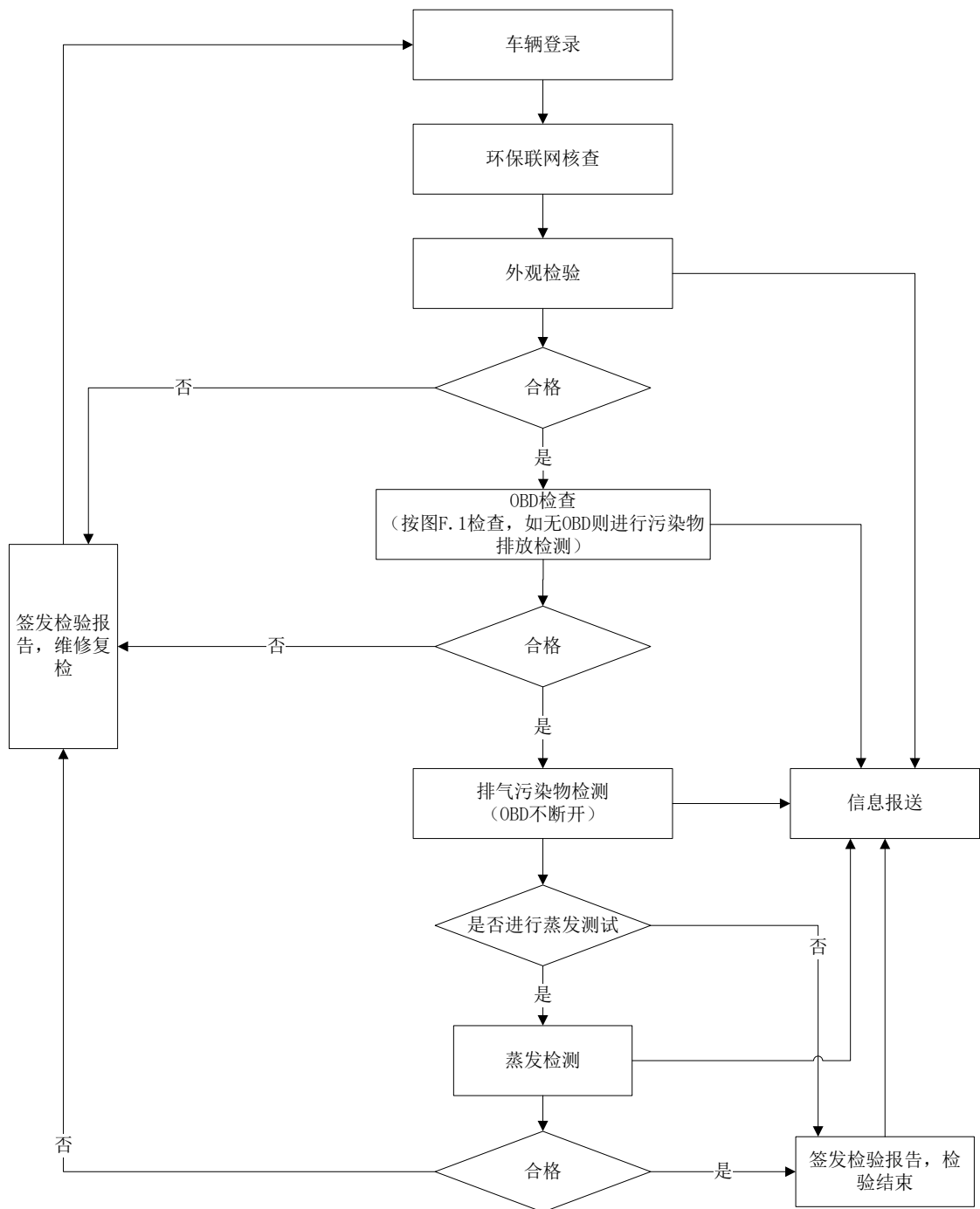
图 3 在用汽车环保检验流程图
