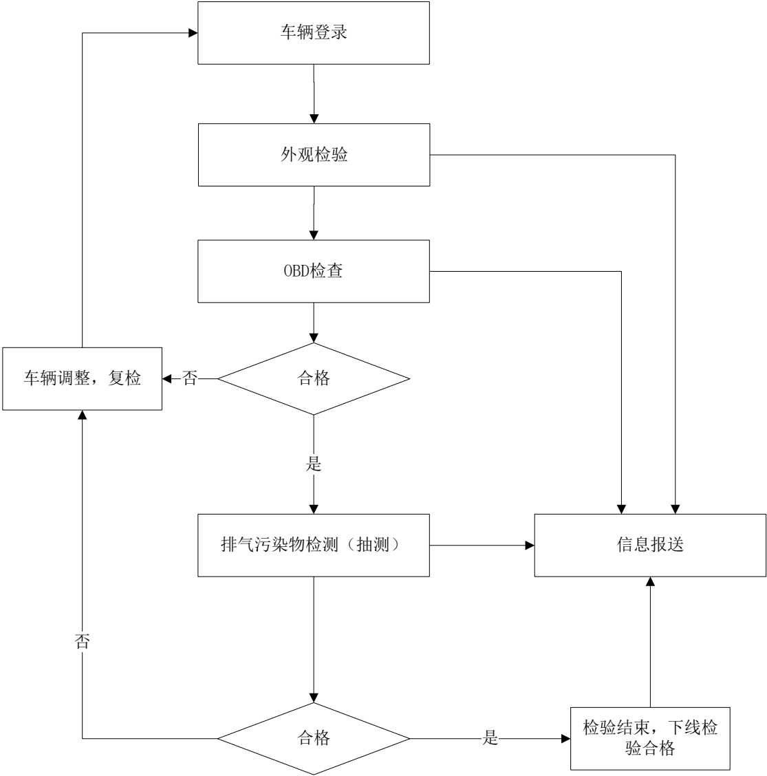
图 1 新车下线环保检验流程图
