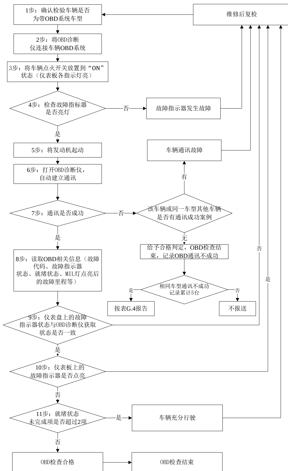
图 F.1 OBD 系统检验流程示意图
