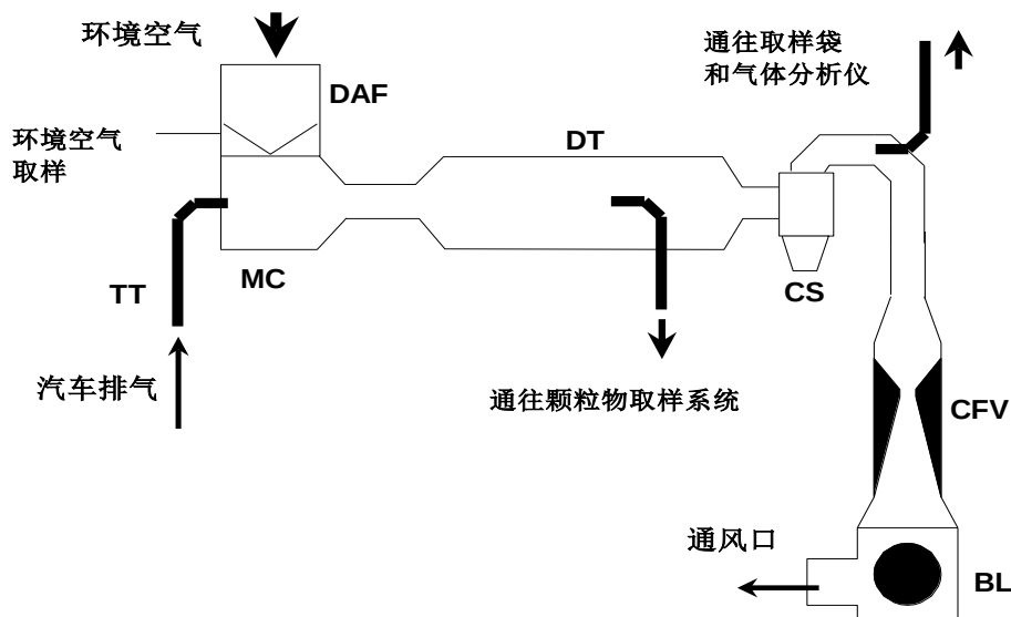
图 C.2 临界流量文丘里管稀释系统
