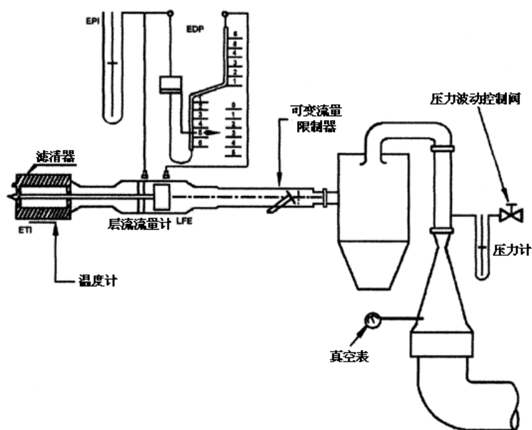
图 C.3 CFV-CVS 检查布置图
