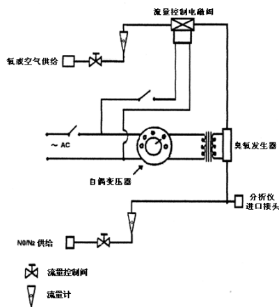
图 C.4 NO x 转化器效率测试装置示意图
