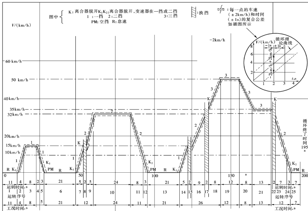
图 C.1 瞬态工况运转循环
